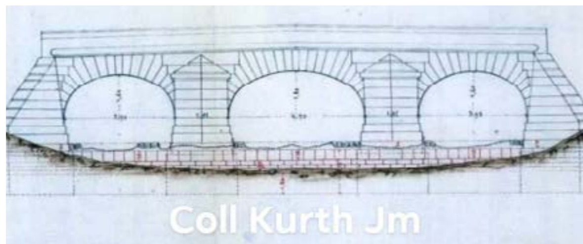
Pont à 3 arches en cintres surbaissés sur le ruisseau de la Bibiche. Longueur : 12,60 m - Largeur : 12 m.
